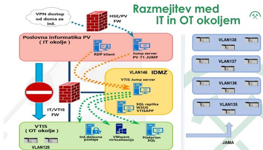
Razmejitev med OT in IT okoljem
