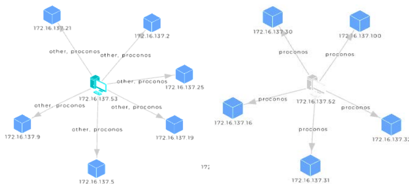
Grafični prikaz poveztivosti SCADE z PLC krmilniki vključno z protokoli
